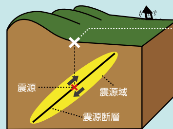
震源等の模式図
